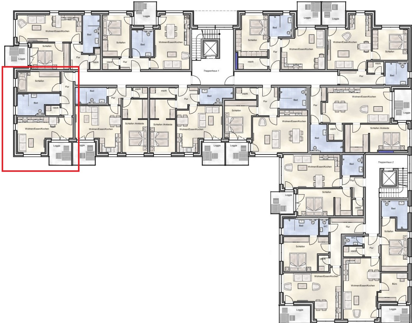
Objekt: Emshouse | Im Hagenkamp 8 in 48282 Emsdetten | 1. Obergeschoss | Wohnung Nr. 3j
